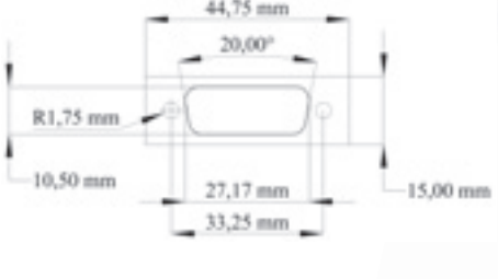
D-Sub 15
