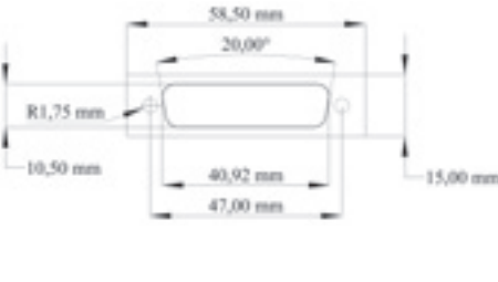
D-Sub 25
