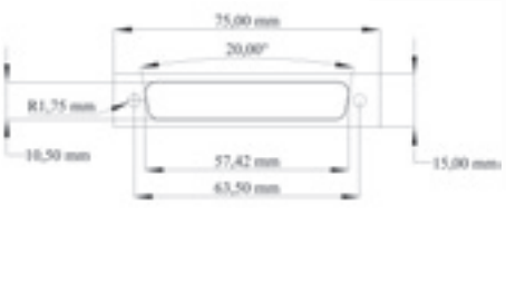
D-Sub 37
