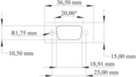
D-Sub 9
